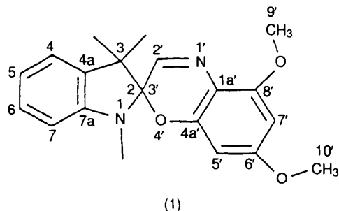
Fig. 1. 5,7-Dimethoxy-1',3',3'-trimethylspiro[2H-1,4-benzoxazine-2,2'-indoline].
